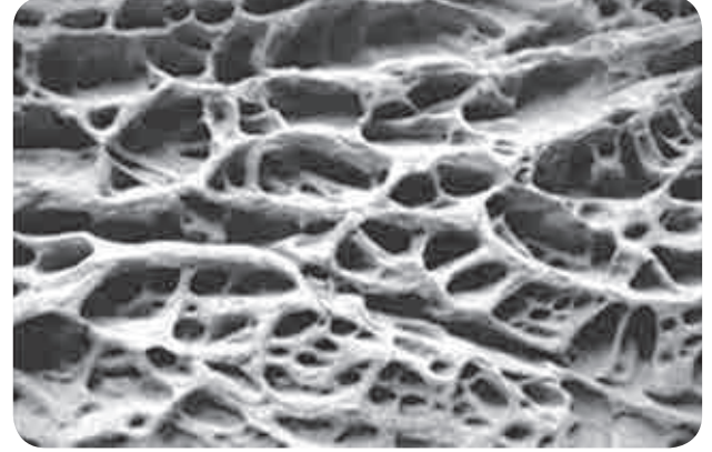
आकृती २.४ : विदारणामुळे मधमाशांच्या पोळ्याप्रमाणे तयार झालेला भू-आकार
