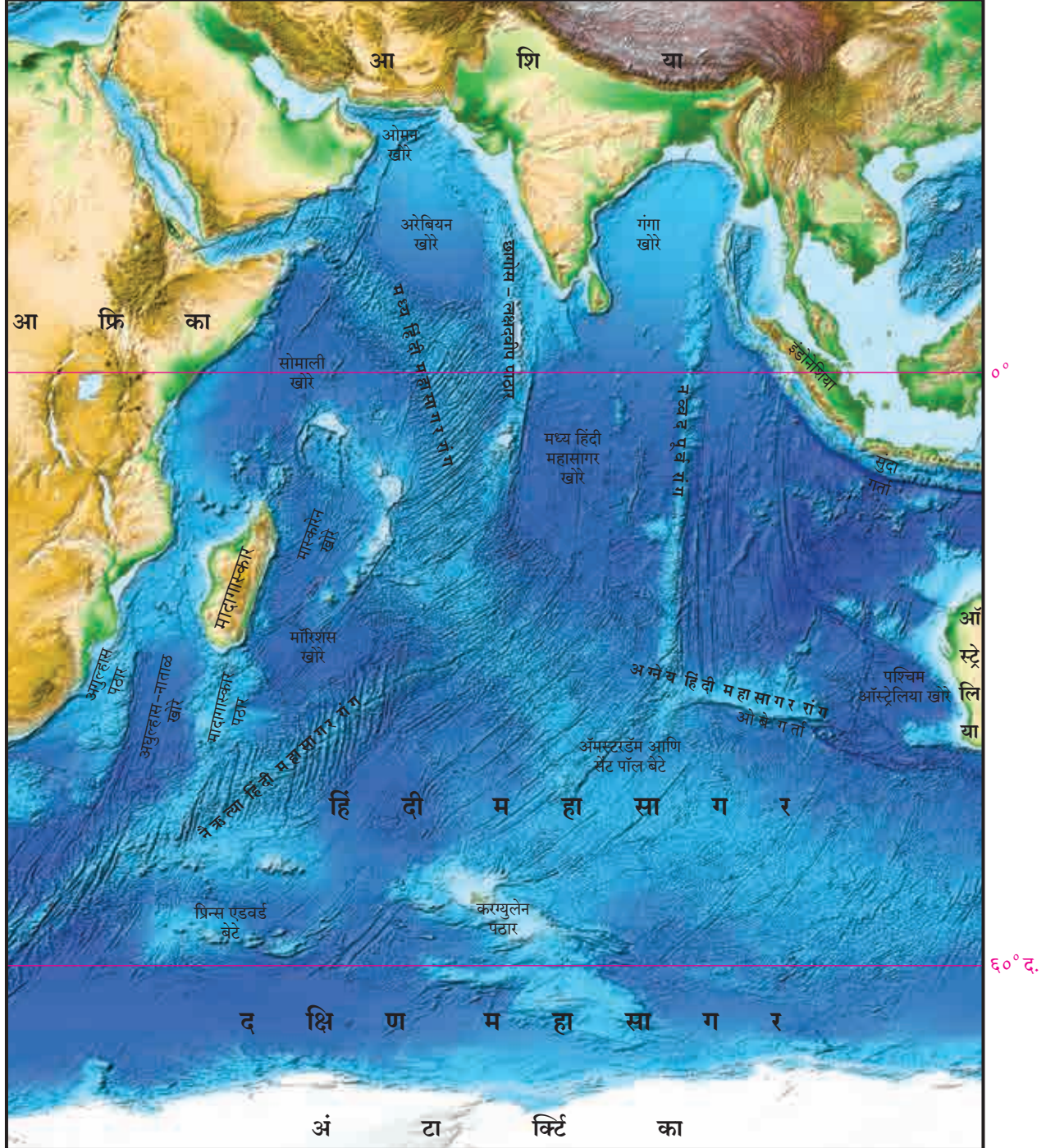
आकृती ७.१ : हिंदी महासागर तळरचना
