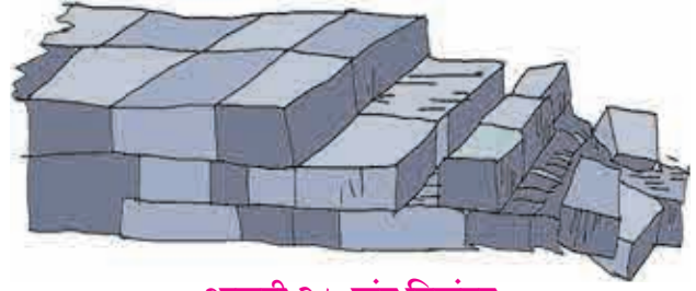
आकृती २.७ खंड विखंडन
