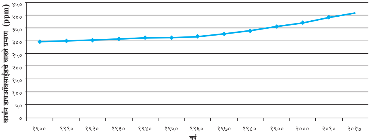
कार्बन डायऑक्साईडचे वाढते प्रमाण (ppm)
