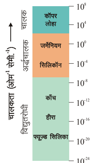
चित्र-6 : पदार्थों की चालकता का बढ़ता क्रम
