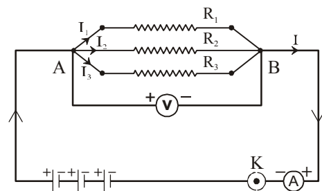
चित्र-8 : समानांतर क्रम में आयोजन
