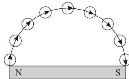
चित्र-1 : चुंबकीय बल रेखा
