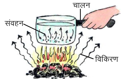
चित्र-4 : ऊष्मा का संचरण तीन प्रकार से हो सकता है।
