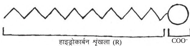
4 (अ) : कार्बोक्सिलेट आयन के भाग
