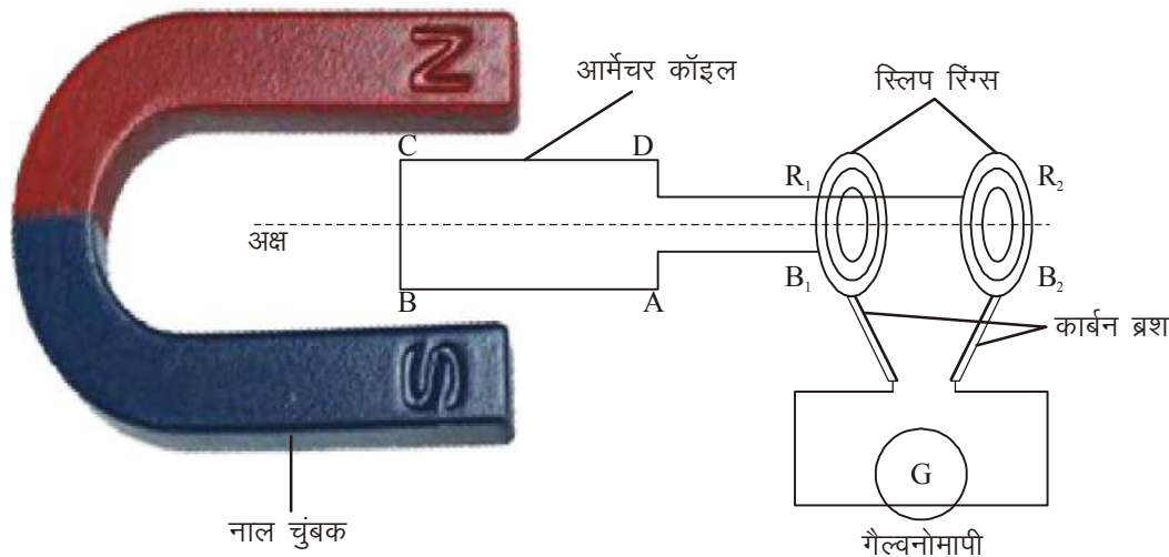
चित्र-16 : विद्युत जनित्र
