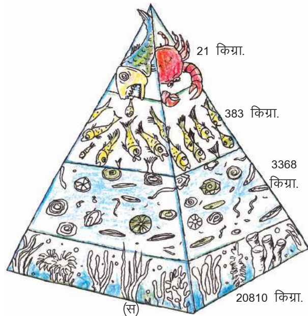
चित्र-9 : जीव भार के पिरामिड (जीव भार प्रति किग्रा./1000 वर्ग मीटर में )
