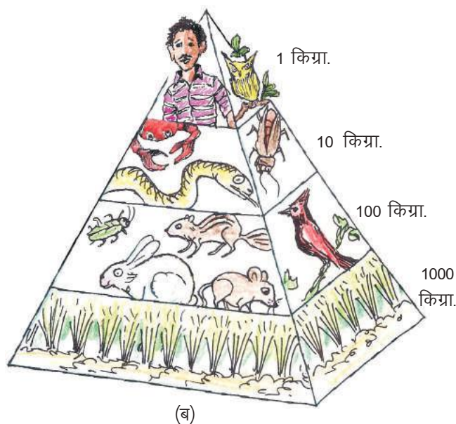
चित्र-9 : जीव भार के पिरामिड (जीव भार प्रति किग्रा./1000 वर्ग मीटर में )
