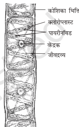
स्पाइरोगाइरा
