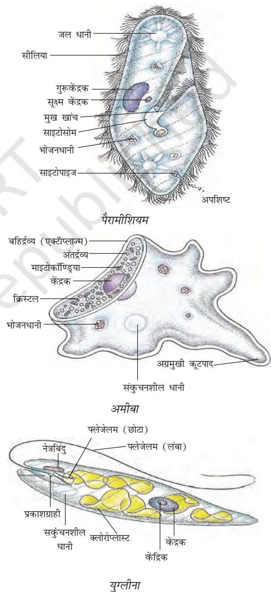
चित्र 7.2: प्रोटोजोआ
